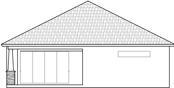
Right Elevation
